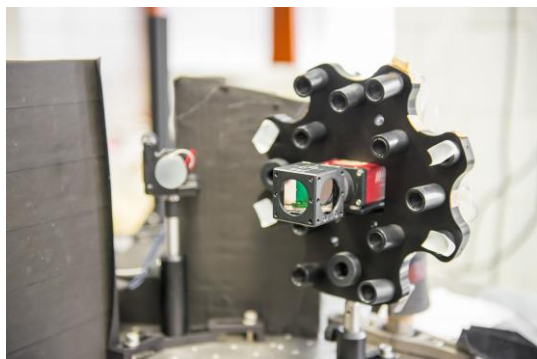
Obr. 2 – vícesměrové holografické měřidlo
